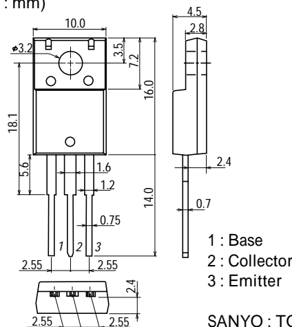
外形図 2041A
